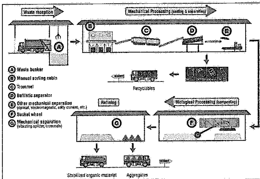
Figura 5. Ilustrimi i Trajtitit Mekanik Biologjik
