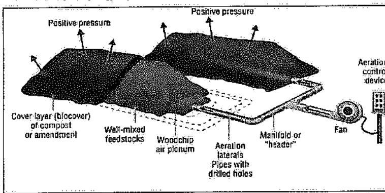
Figura 11. Shembull impianti kompostimi me ajrim të detyruar
