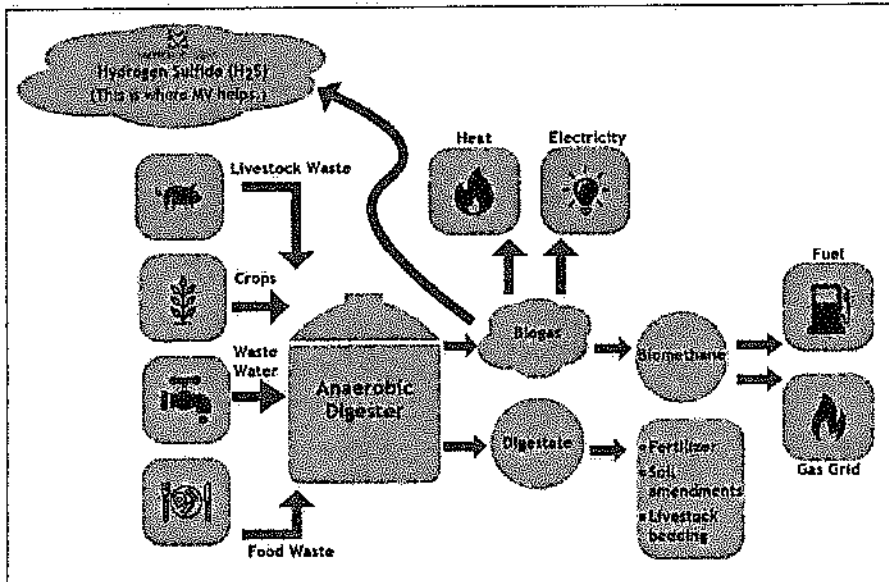
Figura 6. Diagrami i rrjedhës së tretjes anaerobe 6
